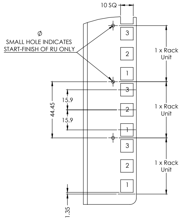
RU PROFILE Rack Unit
